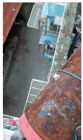
楼顶发生滑移的储水罐。靳方
