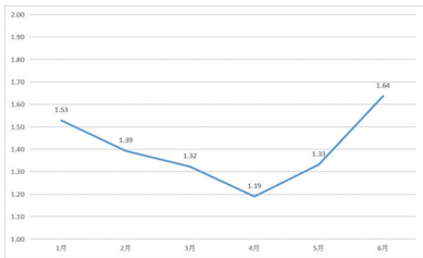
全市电梯困人率变化趋势图
