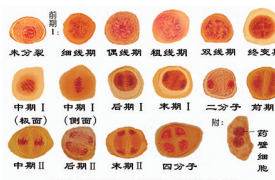
图8 葱兰花粉母细胞减数分裂
