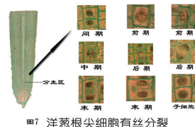
图7 洋葱根尖细胞有丝分裂
