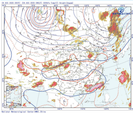
图中588线围起来的区域就是副热带高压。
