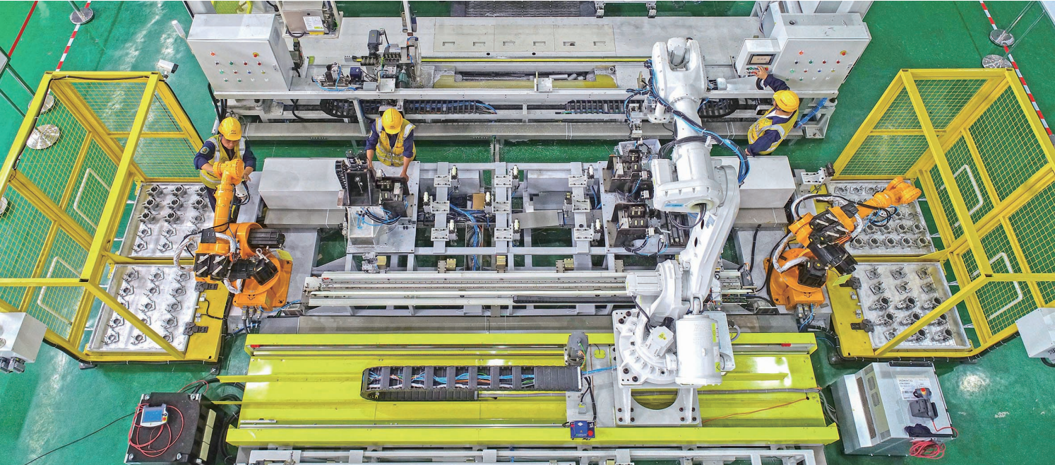
今年5月份，由中国铁建电气化局盐通铁路项目(海安段)投资建设的接触网腕臂自动化预配生产线正式投入使用，能够有效提高盐通高铁接触网工程施工质量和效率，充分满足智能化高铁建设的需求。昨日，工人在生产车间调试设备。姜明摄
