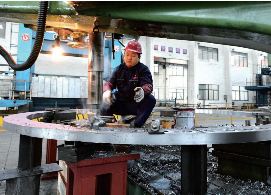
海安高新区的江苏丰禾机械制造有限公司积极融入“一带一路”发展，革新技术、扩展市场，已中标境外8个国家11个水利工程，订单排至明年3月，企业正发动员工加班加点提高产能，争取早日完成在手订单。图为11月24日，工人正在加紧赶制水利水电机械产品。 顾华夏 张加斌摄
